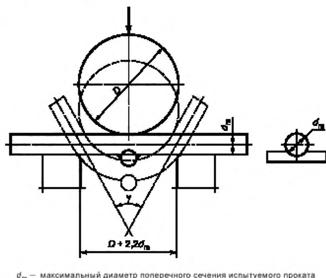
Рисунок Г.1 — Схема испытаний на изгиб крестообразных сварных соединений
